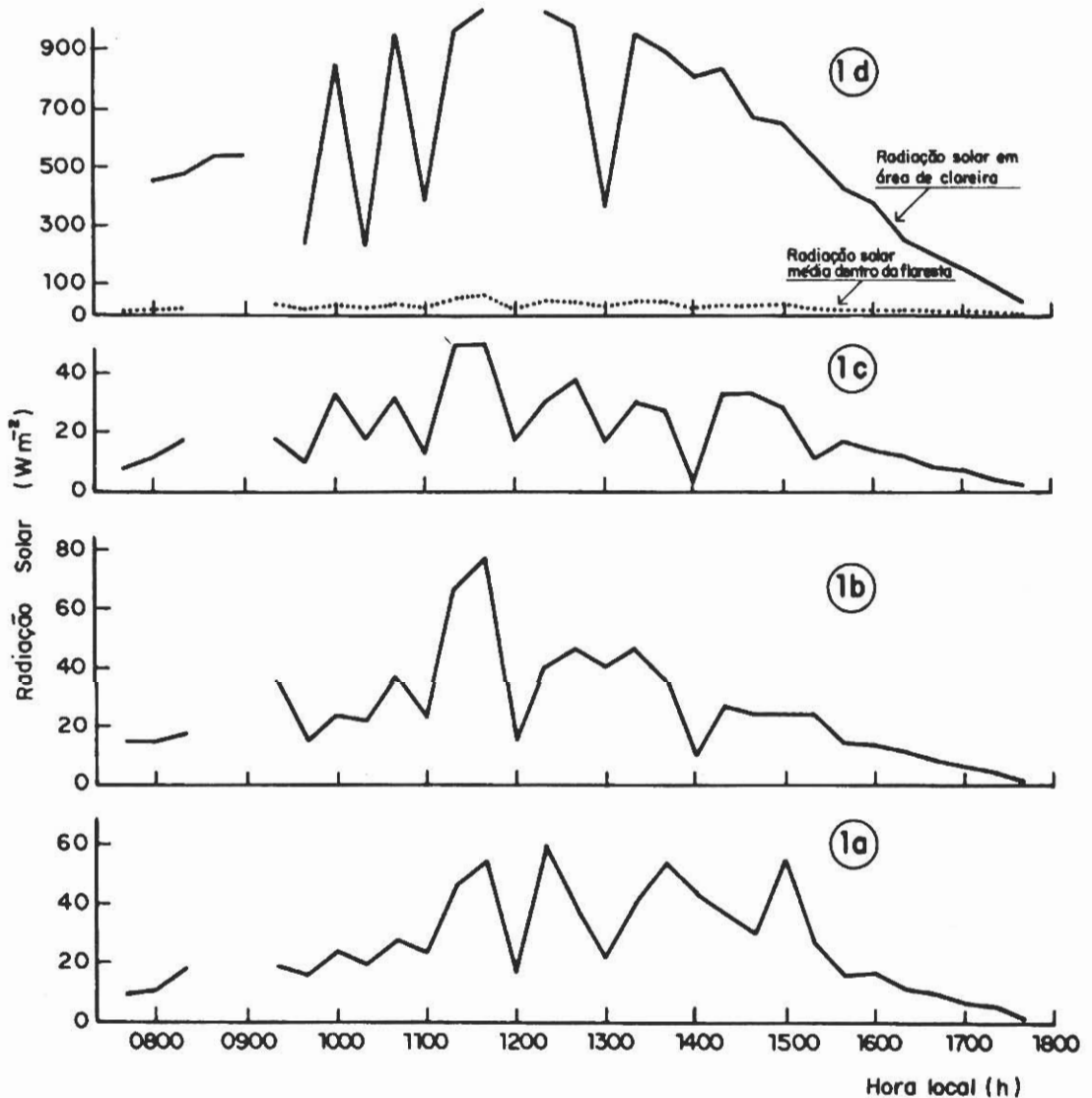
Fig. 1. Distribuição da radiação solar em função da hora local para 3 piranômetros instalados dentro da floresta (1a, 1b., 1c) e um situado em área aberta (1d). A radiação média para os 3 sensores da mata é apresentado em 1d. Medidas feitas em 07.11.86 em Tucuruí/PA.
